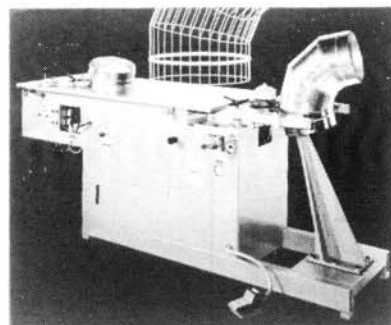
エルボ加工機(ゴアロッカー)
